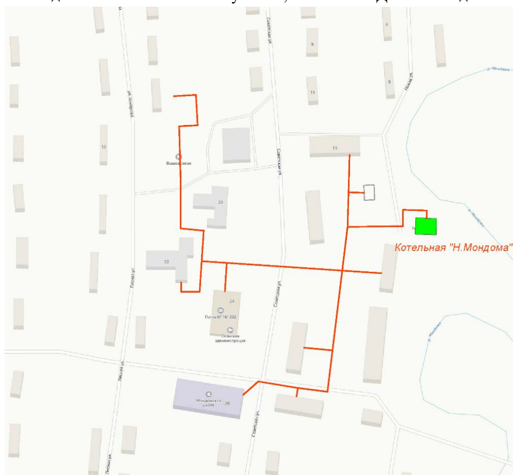
Рис.2.10 – Зона действия котельной «Н.Мондома»
