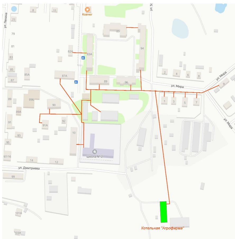
Рис.2.1 – Зона действия котельной «Агрофирма»
