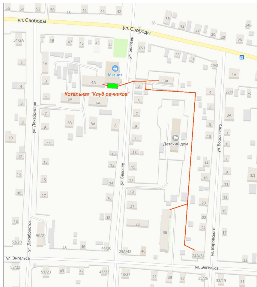
Рис.2.5 – Зона действия котельной «Клуб речников»
