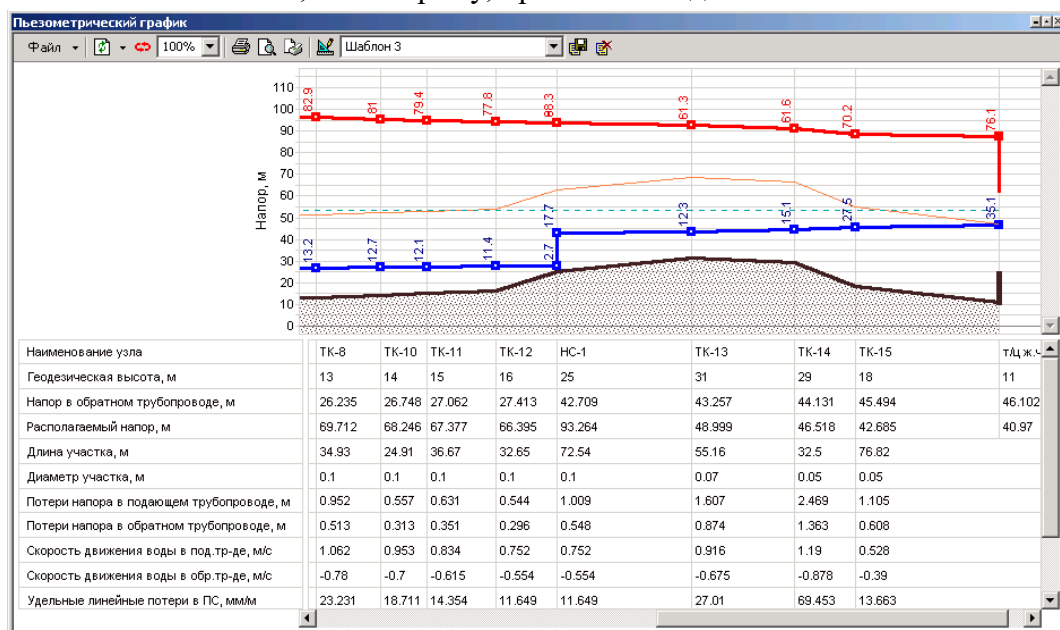
Рисунок 14.1. Пример пьезометрического графика
